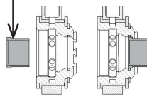
Kühlscheibe KS
