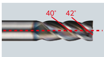
不等リード Unequal Helix Angle
