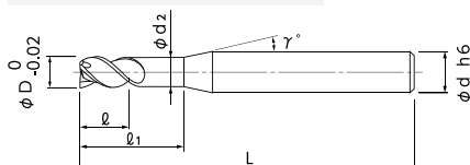
形状 B：ロングネックタイプ TYPE B: Long neck Type
